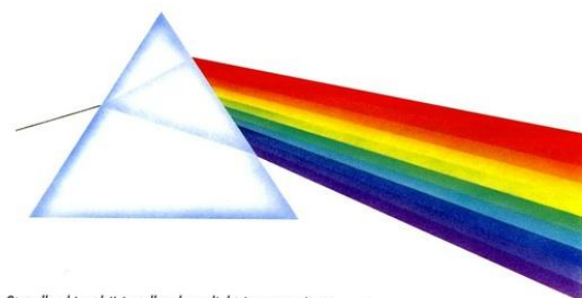
Straalbreking bij invallend zonlicht in een prisma
