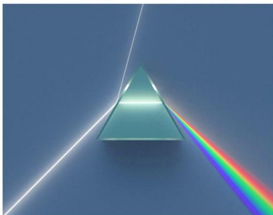
Foto: Straalbreking van wit licht door een prisma
